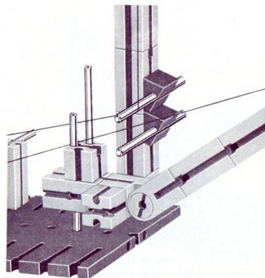
Bild 60.1 Seilführung
